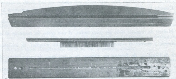
3 Peigne pour denteler les timbres en feuilles.
